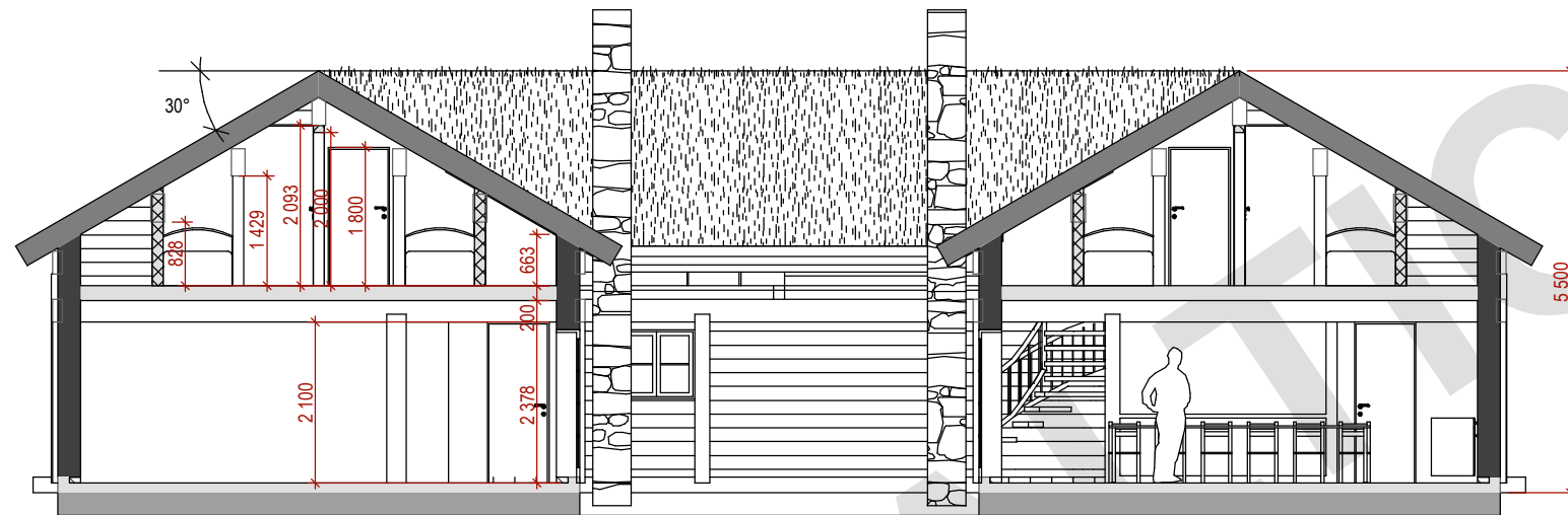
SNITT A-A
