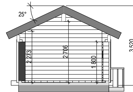
SNITT C-C
