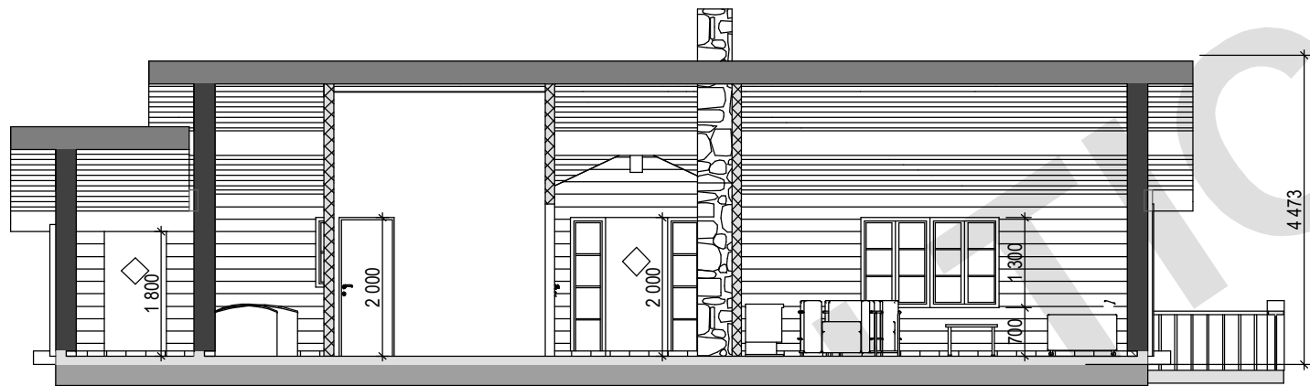
SNITT A-A
